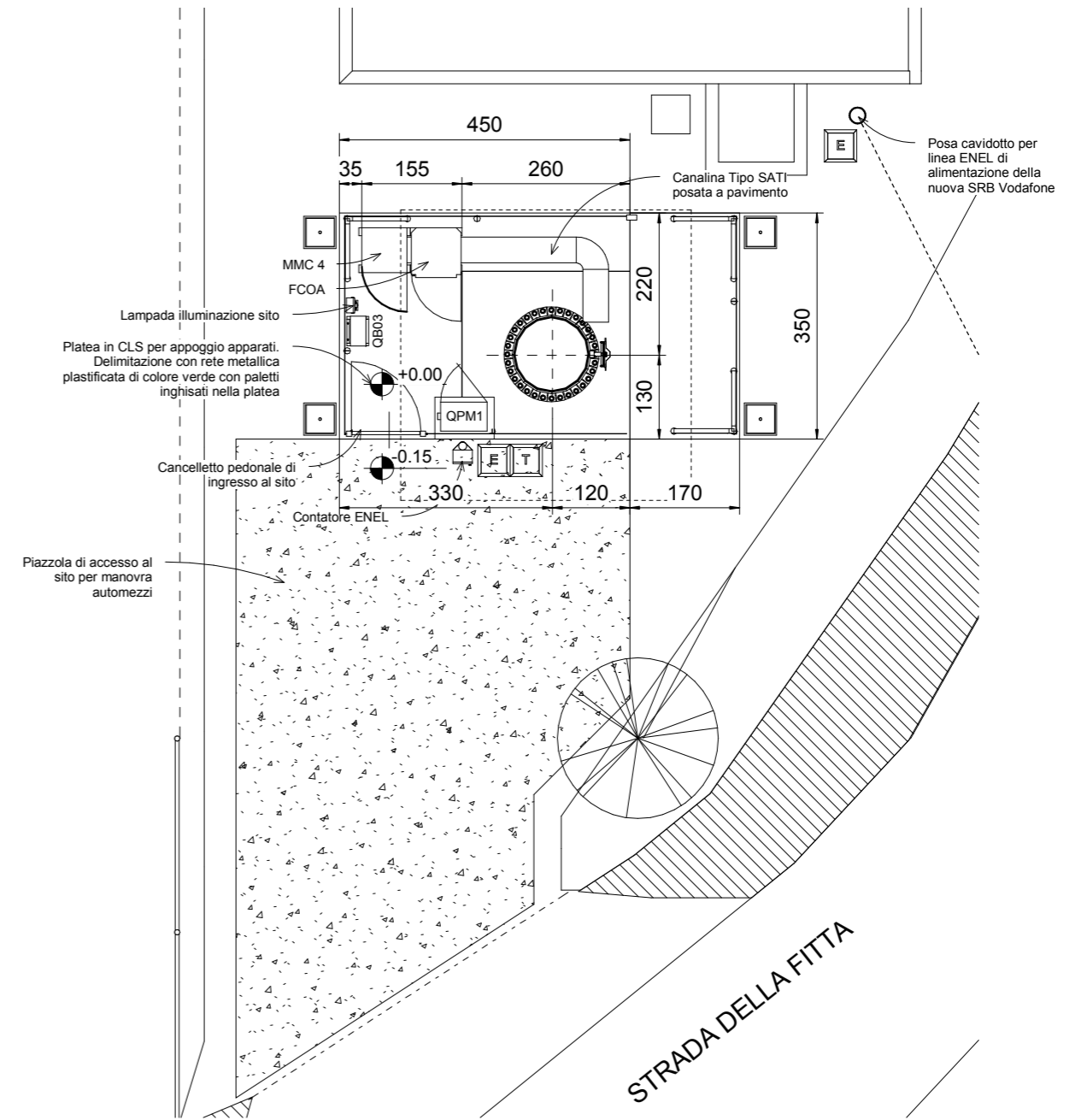
DETTAGLIO PIANTA (1:100)
